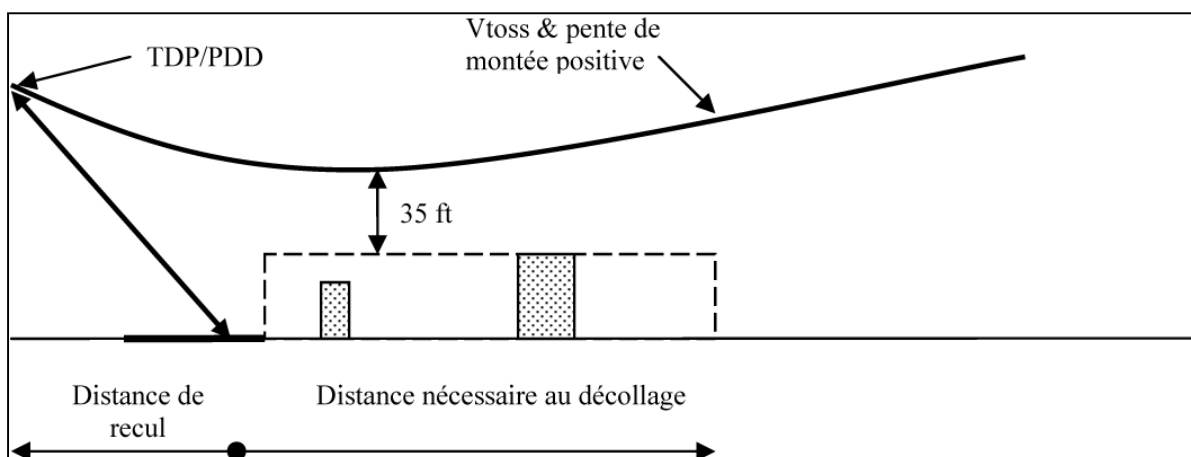
Figure 3. – Décollage d'une hélistation
