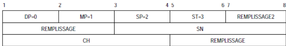
Figure 5-18. Paquet CONFIRMATION DE RÉINITIALISATION
