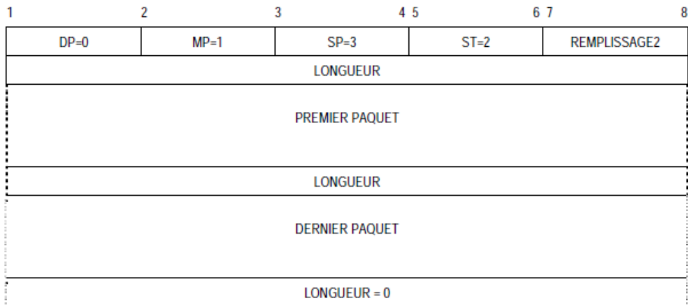
Figure 5-20. Paquet MULTIPLEXÉ
