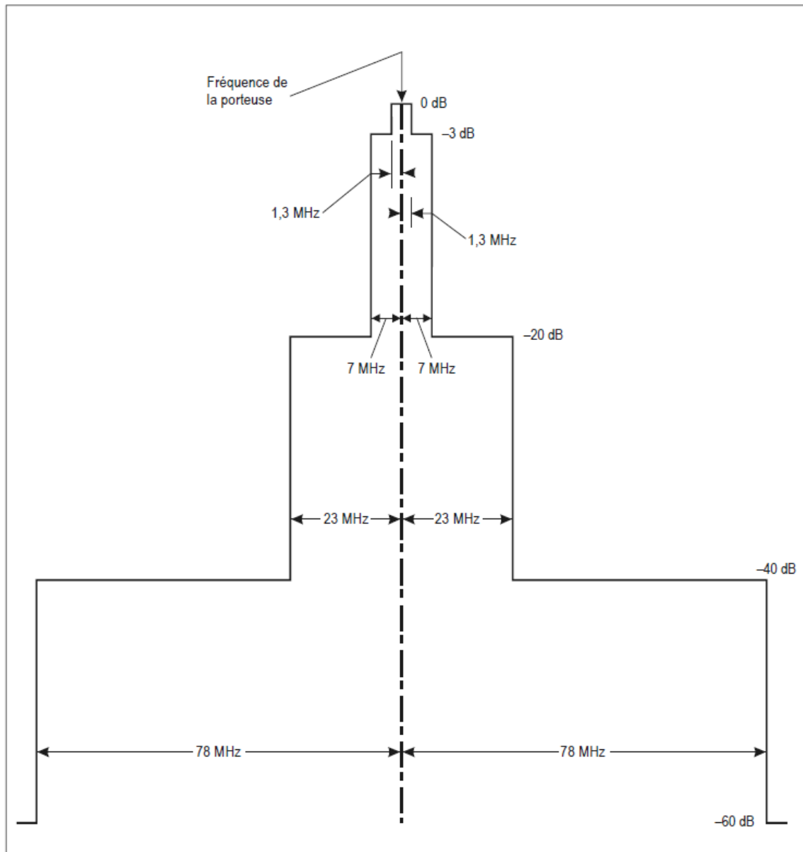
Figure 3-5. Limites du spectre pour le transpondeur
