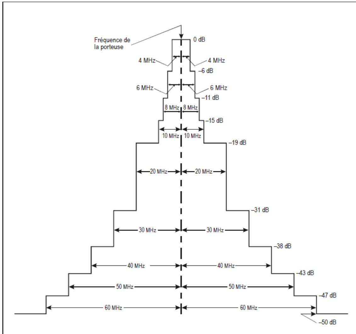
Figure 3-2. Limites du spectre pour l'interrogateur
