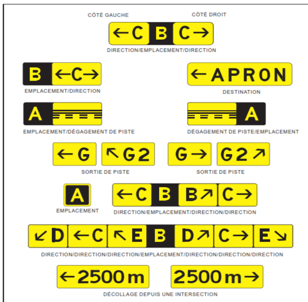
Figure 5-30. Panneaux d'indication
