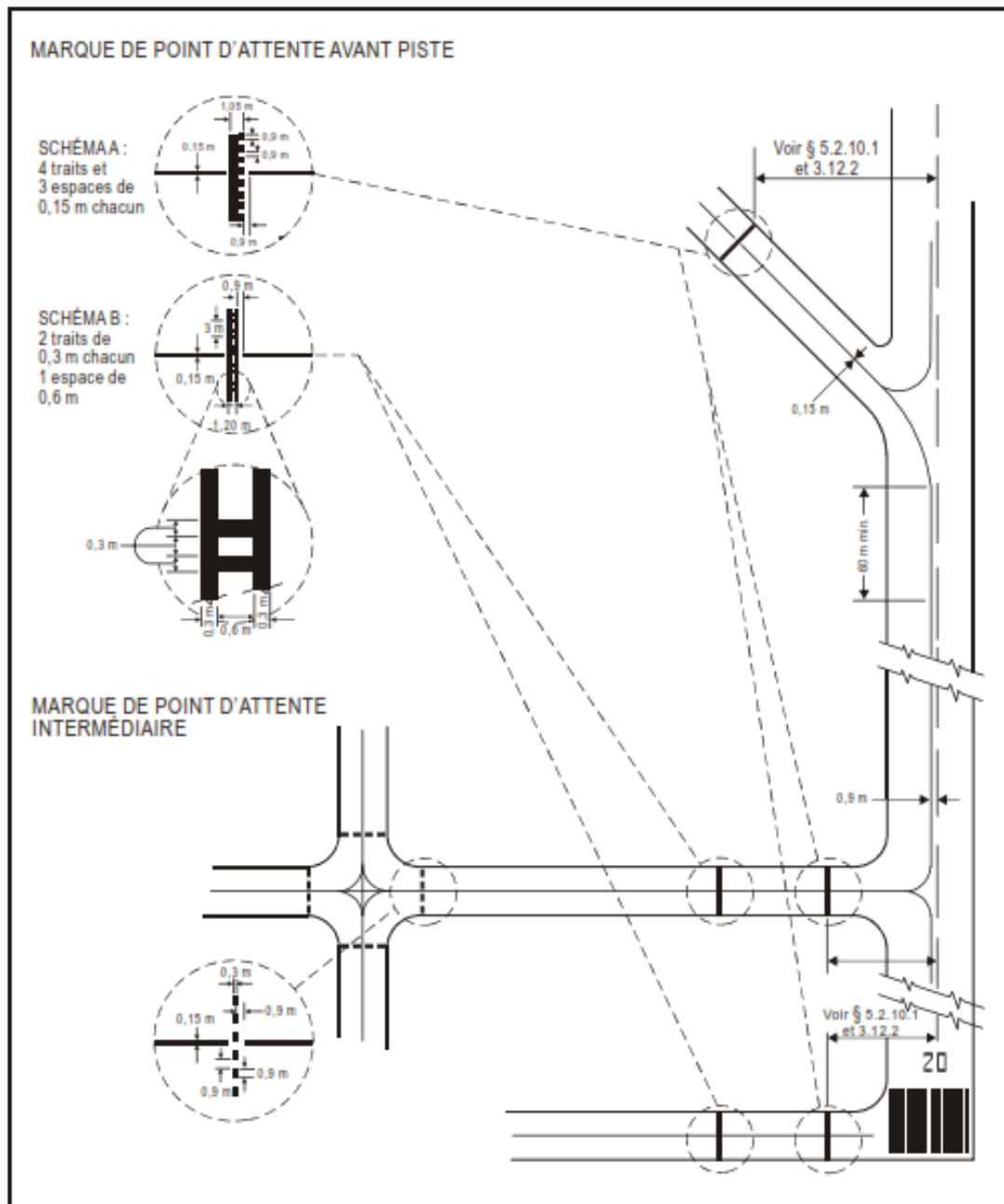
Figure 5-6. Marques de voie de circulation
