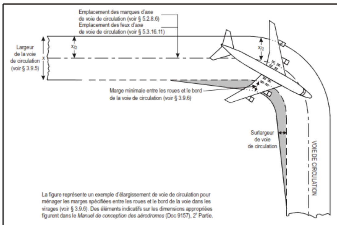
Figure 3-2. Virage de voie de circulation
