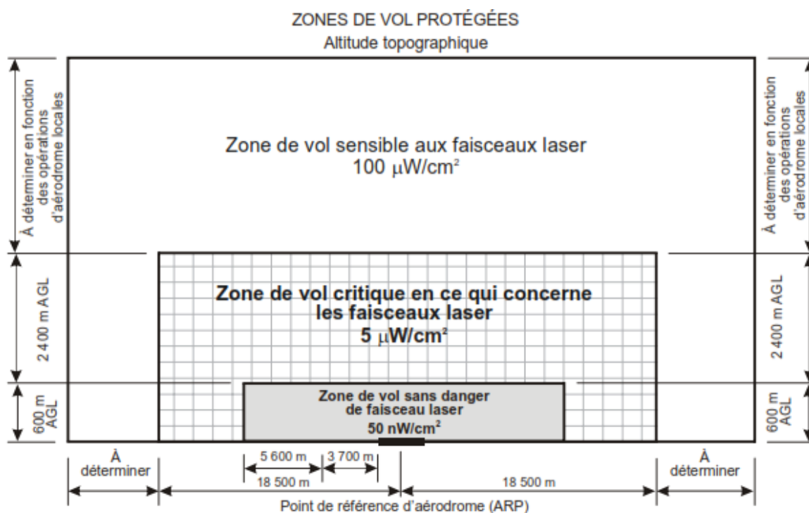
Figure 5-13. Zones de vol protégées avec indication du niveau maximal d'éclairciment énergétique des faisceaux laser visibles
