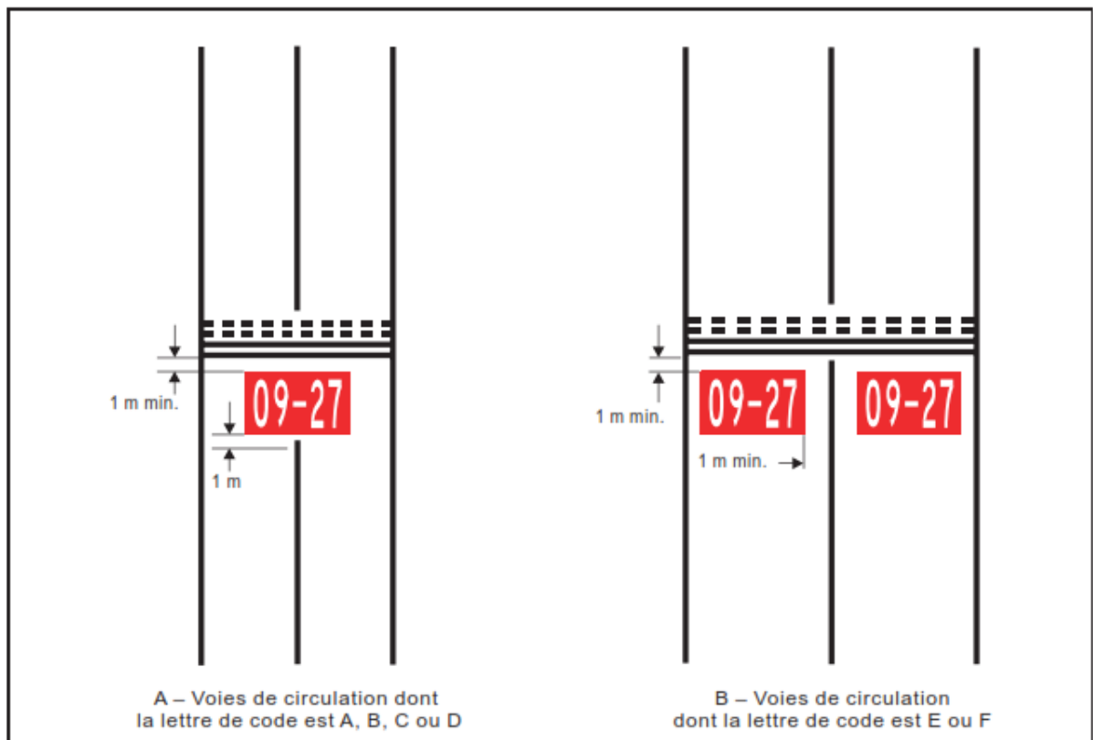
Figure 5-10. Marque d'obligation
