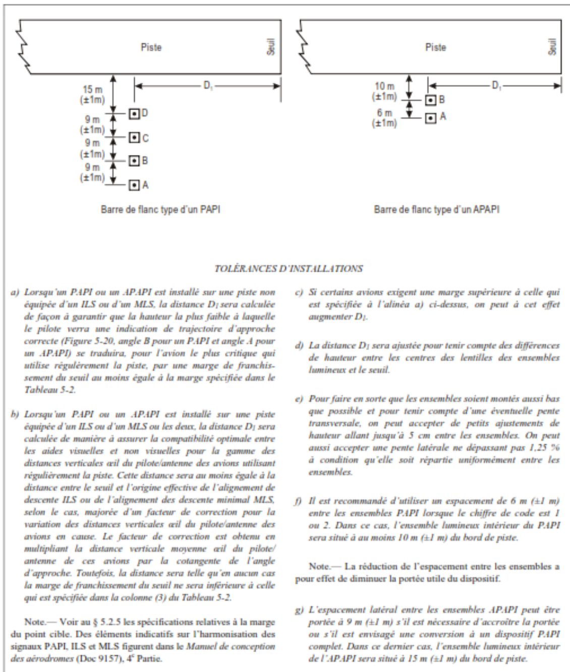
Figure 5-19. Implantation du PAPI et de l'APAPI
