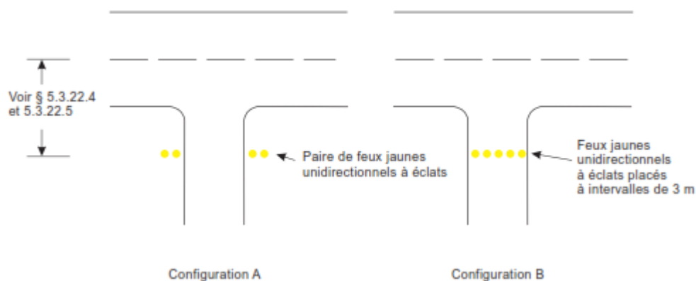
Figure 5-28. Feux de protection de piste
