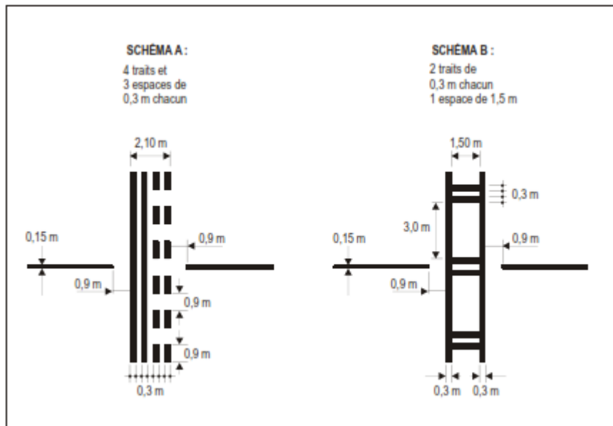
Figure 5-8. Marques de point d'attente avant piste
