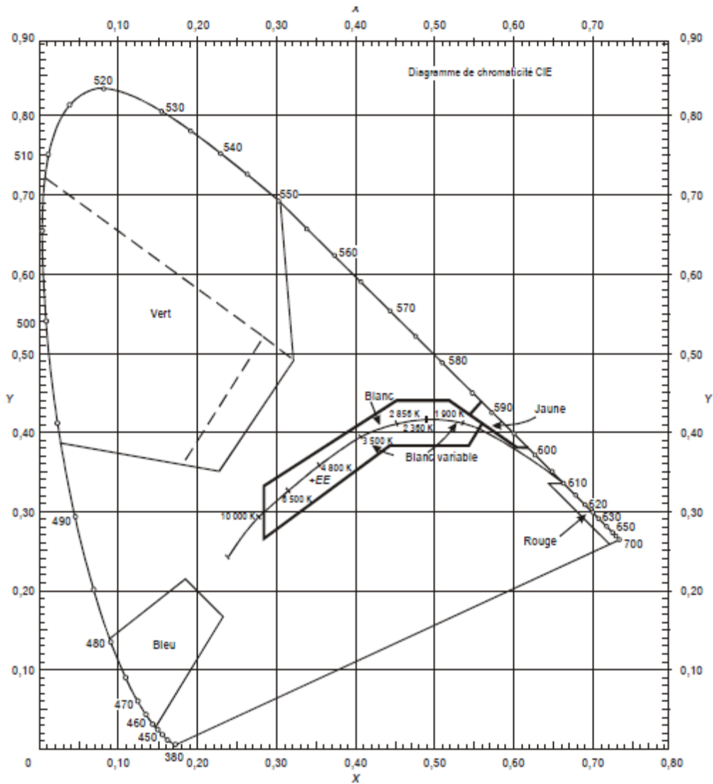
Figure A1-1. Couleurs des feux aéronautiques à la surface
