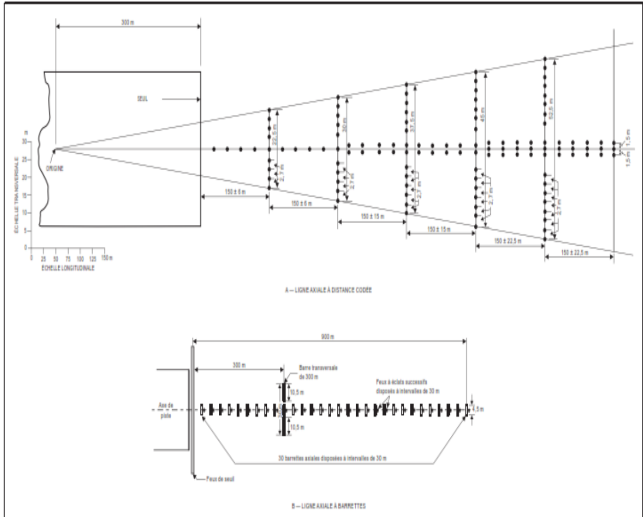
Figure A-8. Dispositif lumineux d'approche de précision de catégorie I
