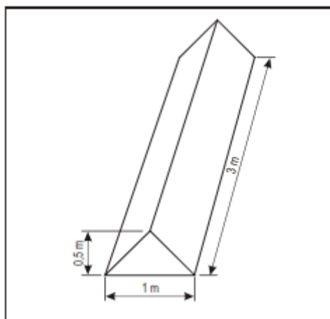
Figure 5-33. Balise de délimitation
