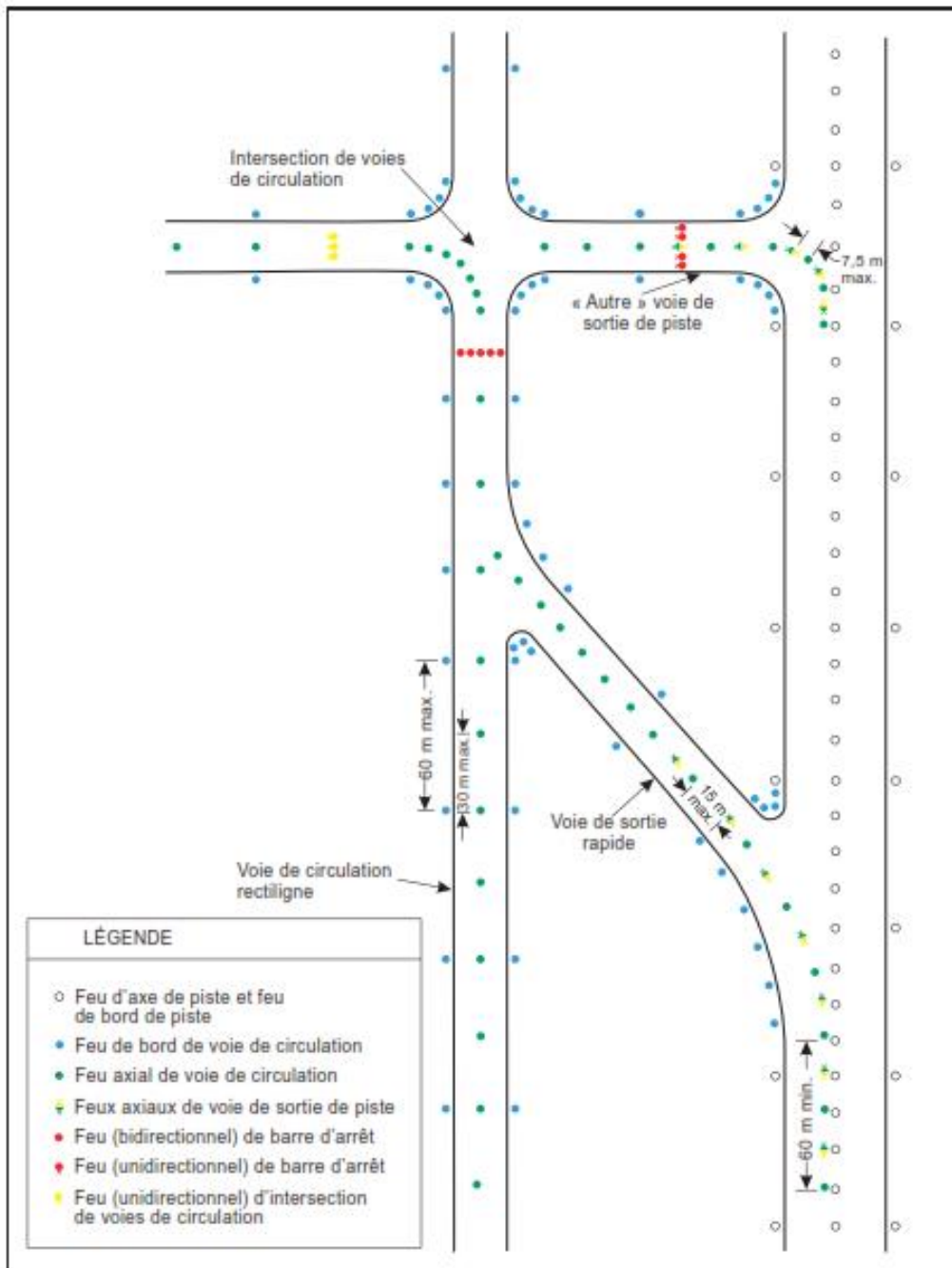
Figure 5-26 Balisage lumineux de voie de circulation
