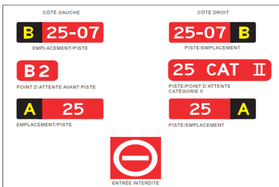
Figure 5-29. Panneaux d'obligation
