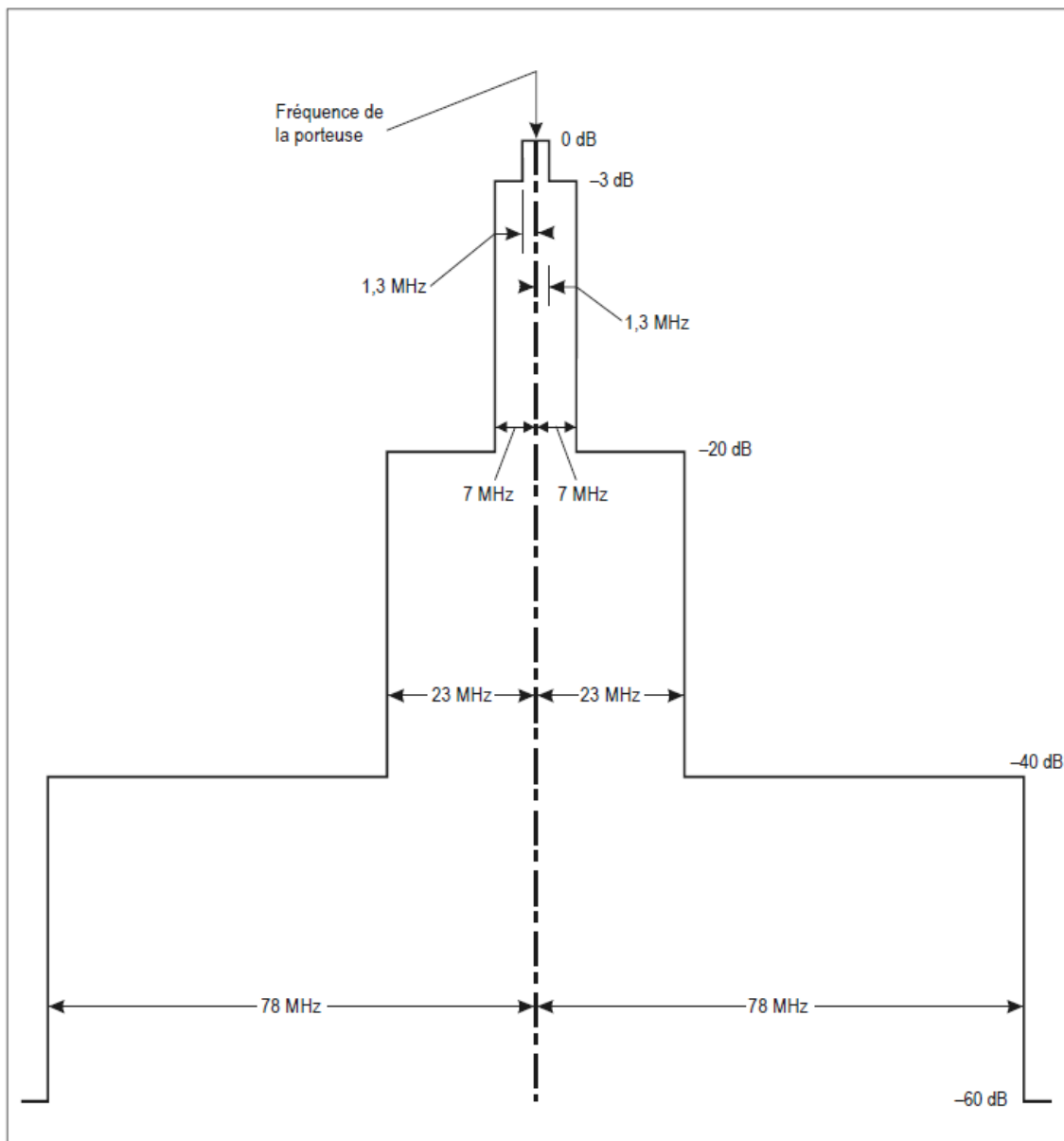
Figure 3-5. Limites du spectre pour le transpondeur
