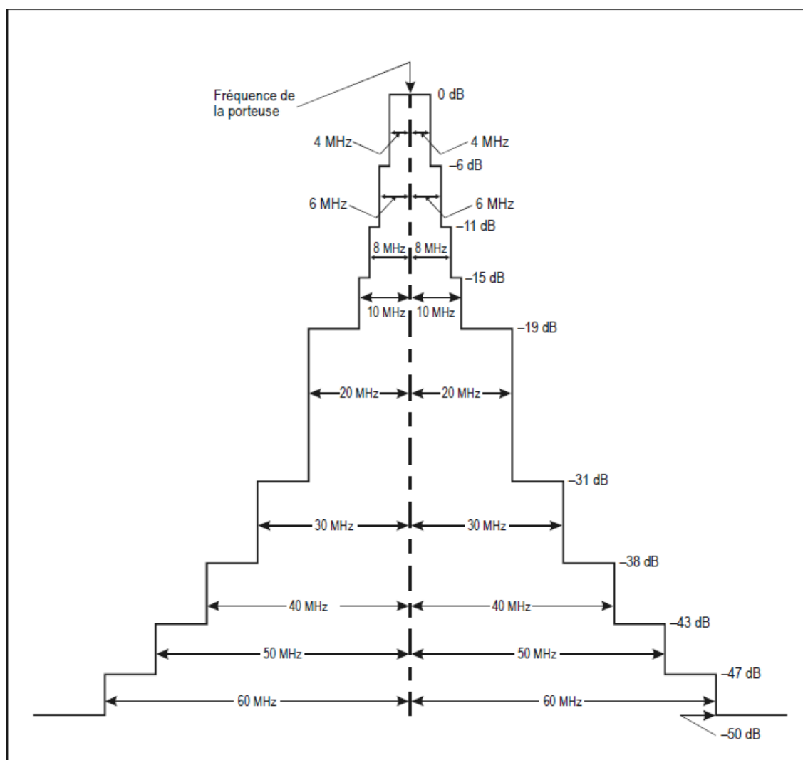
Figure 3-2. Limites du spectre pour l'interrogateur
