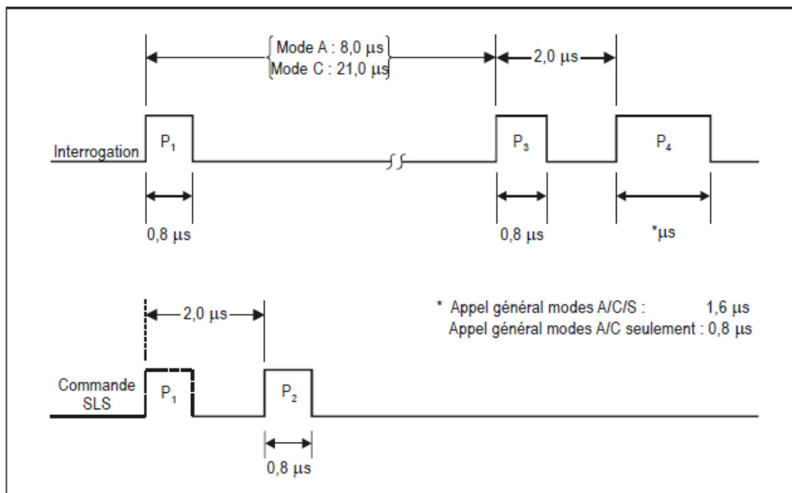
Figure 3-3. Séquence d'impulsions d'interrogation intermodes
