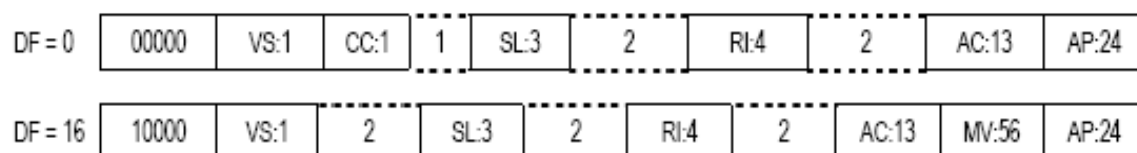
Figure 4-1. Formats de surveillance et de communication utilisés par l'ACAS
