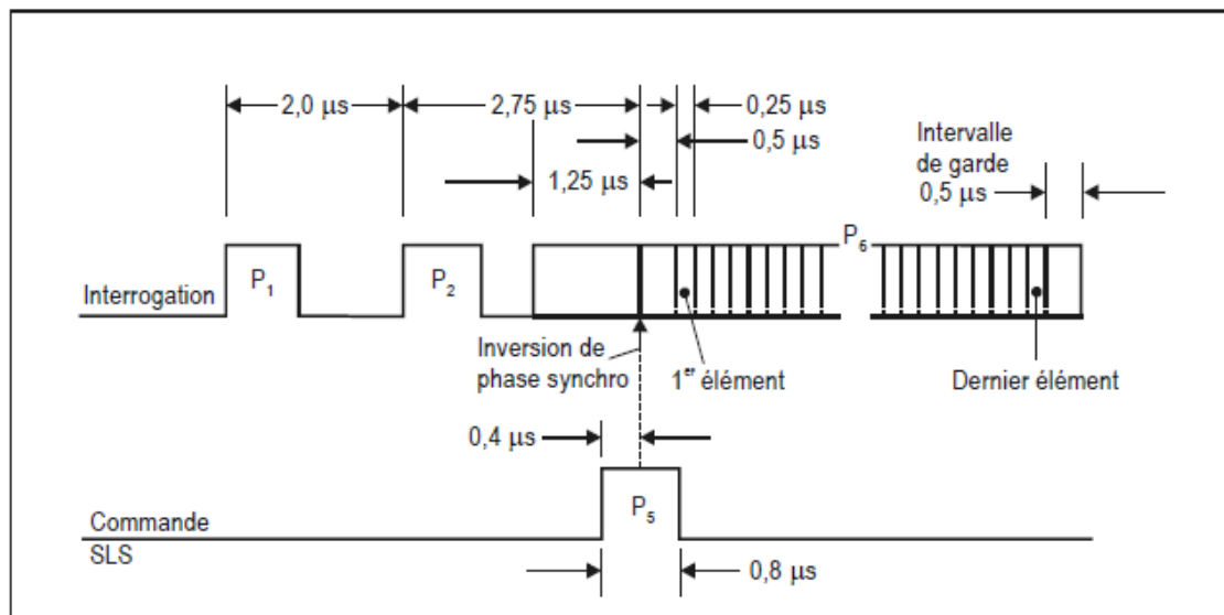
Figure 3-4. Séquence d'impulsions d'interrogation mode S
