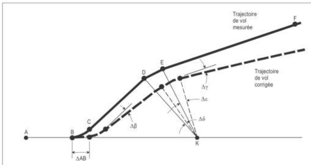
Figure A1-4. Profil de décollage mesuré
