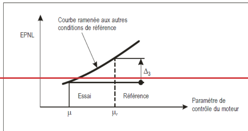
Figure A2-12. Ajustement au bruit à la source
