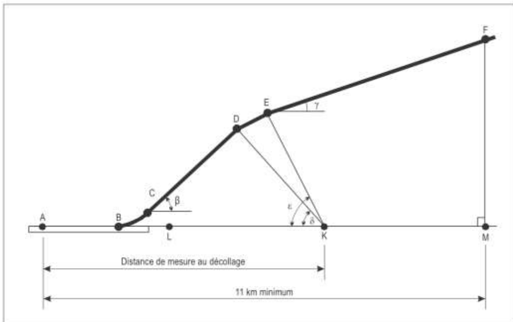
Figure A1-4. Profil de décollage mesuré
