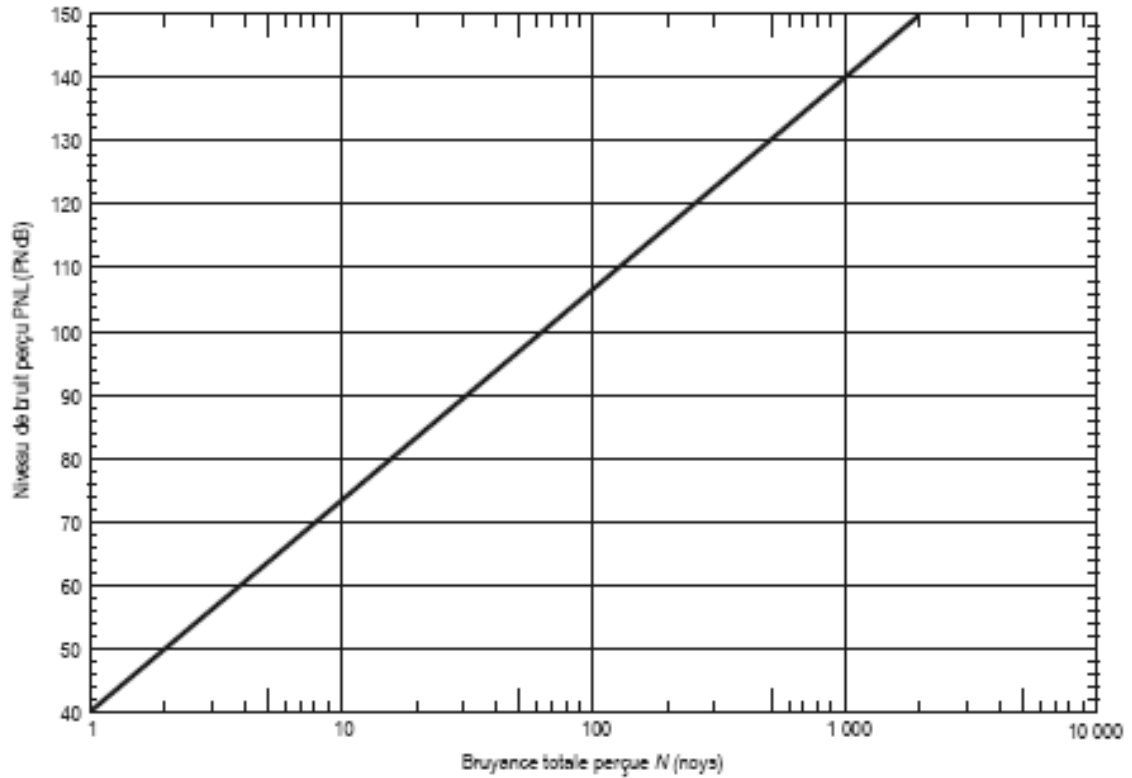
Figure A1-1. Niveau de bruit perçu en fonction de la bruyance totale perçue
