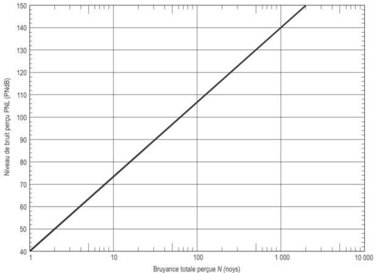
Figure A1-1. Niveau de bruit perçu en fonction de la bruyance totale perçue
